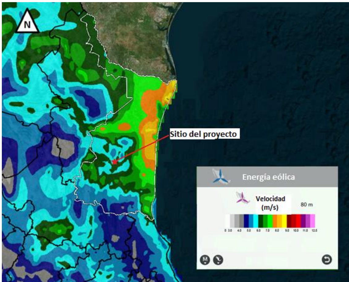
Figura 6 POTENCIAL DEL RECURSO EÓLICO EN MÉXICO
