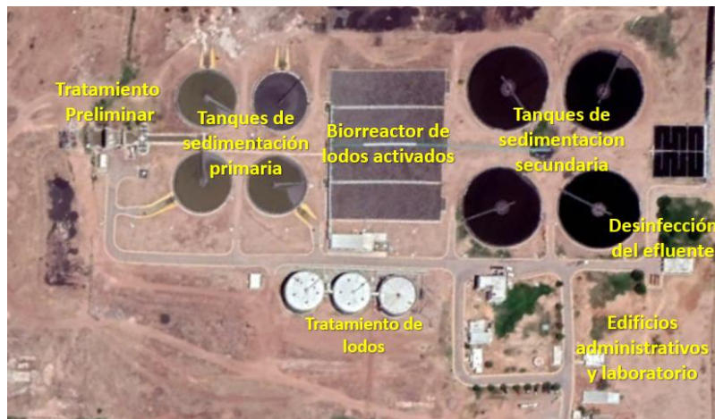
Figura 4 PTAR SUR. PROCESO DE TRATAMIENTO
