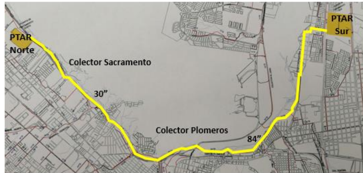
Figura 2 SISTEMA DE CONDUCCION POR GRAVEDAD
